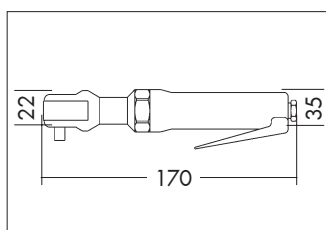
Abmaße 1/4"- und 3/8"-Variante
